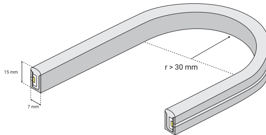
Rys.2. Rysunek poglądowy minimalnego promienia gięcia.
