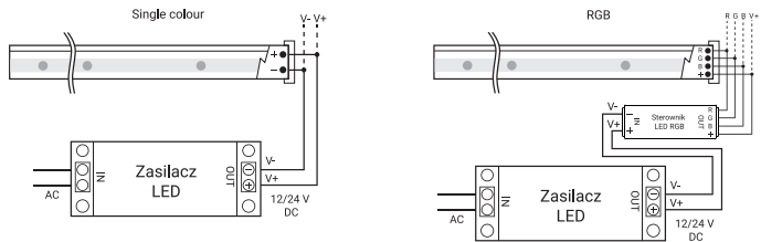
Rys.3. Schemat prawidłowego podłączenia taśmy do zasilacza.
