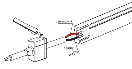
Zaaplikować silikon do wnętrza końcówki zasilającej oraz na brzegi otoku, następnie nasunąć przyłącze na otok.
