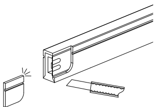
Należy odciąć 3 mm silikonowego otoku, tak aby odsłonił wbudowaną taśmę LED.
