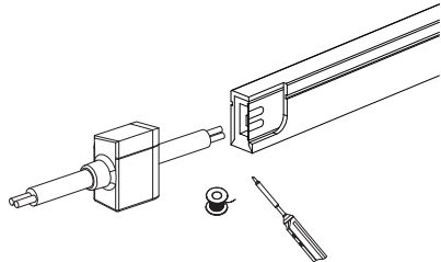
Przylutować kable zgodnie z oznaczeniami na taśmie LED.
