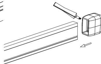
Zaaplikować silikon do wnętrza zaśleпки a następnie nasunąć ją na brzeg otoku.
