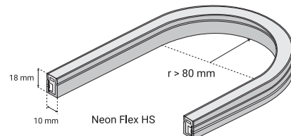
Rys.2. Rysunek poglądowy minimalnego promienia gięcia.
